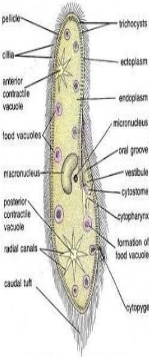
Fig. 20.1. Paramecium caudatum .
